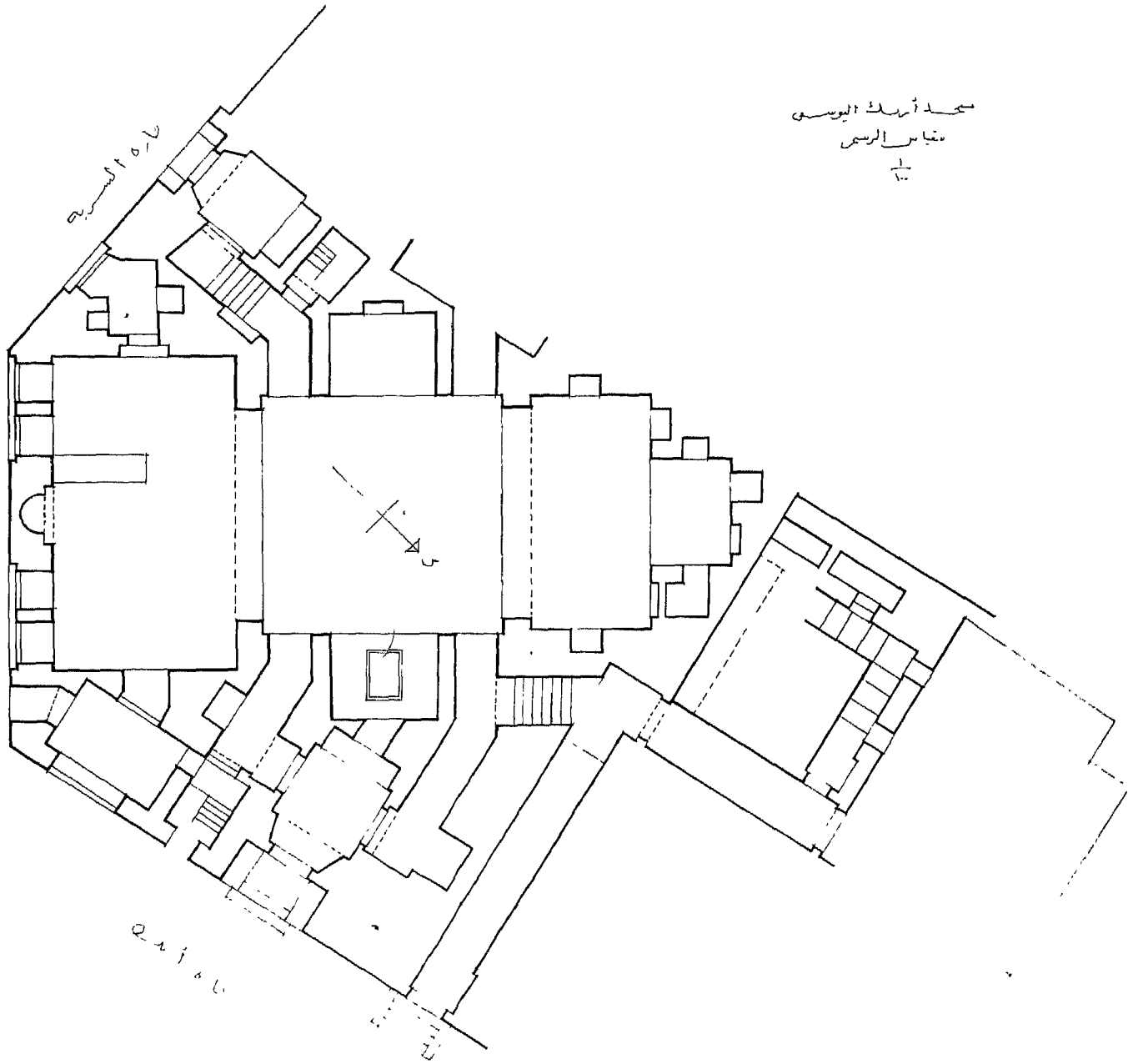
شكل (١٢) يبين مسقط أفقى لمدرسة أزيك اليوسفي بحى طولون بالسيدة زينب رضوان الله عليها
